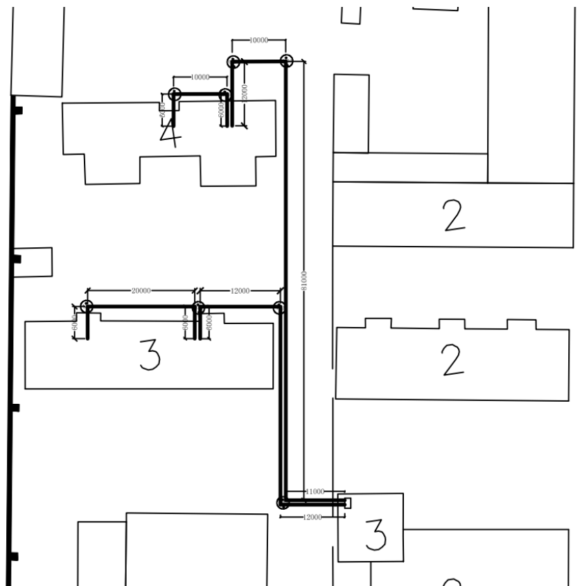
施工简图
